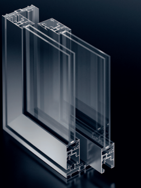
Schuifdeur Schüco ASS 50 Coulissant Schüco ASS 50
